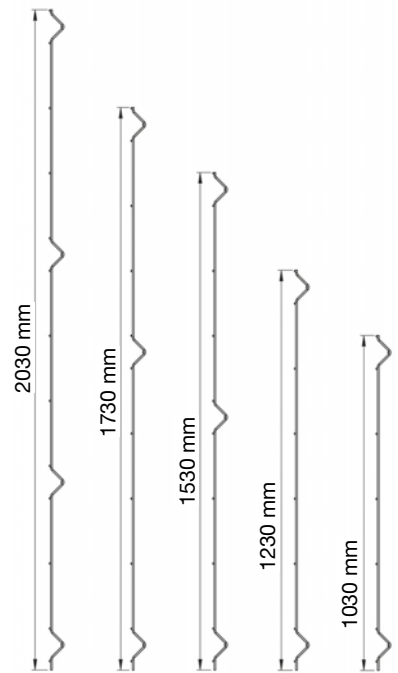
Standardhöhen und Sickenanzahl
