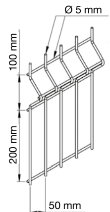
Standardmasche und Drahtstärke
